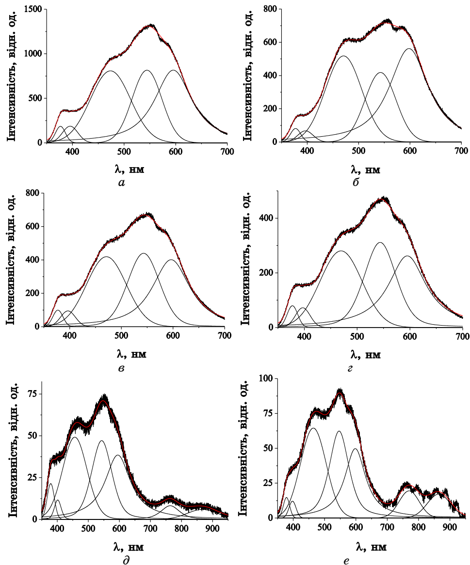
Рис. 2. Розклад спектрів фотолюмінесценції з використанням Гауссових кривих для чистого ПТФЕ ( a ) та його наноккомпозитів із 0,1 ( b ), 0,5 ( c ), 1,0 ( d ), 2,0 ( e ), 5,0 ваг.% БСВНТ ( e ). 2
