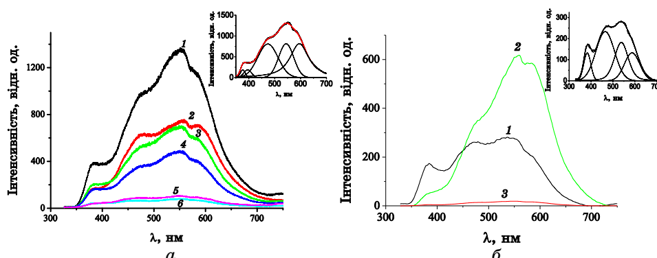
Рис. 1. Спектри фотолюмінесценції: а) поліетилену (1) та композитів ПЕ-БСВНТ з 1,0 (2) та 2,0 (3) об.% БСВНТ; б) чистого політетрафторетилену (1) та його нанокompозитів з 0,1 (2), 0,5 (3), 1,0 (4), 2,0 (5), 5,0 ваг.% (6) БСВНТ (температура T = 300 К, довжина хвилі збудження \lambda_e = 325 нм). 1
