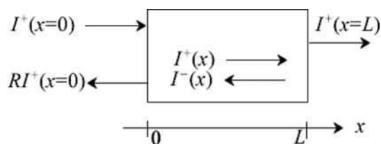
Рис. 7. К выводу связи между коэффициентом прохождения и средней длиной свободного пробега на примере однородного 1D-проводника. 7
