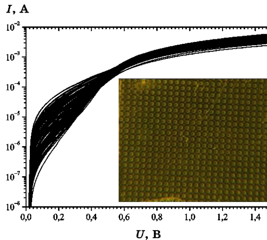
Рис. 1. ВАХ контактів з бар'єром Шотткі Au-TiB x -n-GaN, зібрані з контактів по усій пластині; на вставці — зовнішній вигляд тестової пластини. 1
