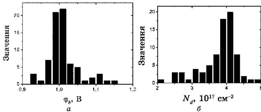
Рис. 7. Гістограми розподілу висоти бар'єру Шотткі (а) та N_d (б) по пластині, одержані з ВФХ. 7
