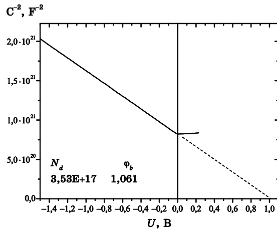
Рис. 6. ВФХ діоди Шотткі Au-TiB x -n-GaN, ВАХ якої представлено на рис. 2. 6
