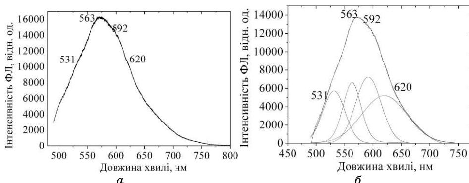
Рис. 6. Спектри фотолумінесценції ПВХ (а) при температурі і 293 К та його розклад на компоненти (б) ( \lambda_{\text{зб}} = 488 \text{ нм} ).
