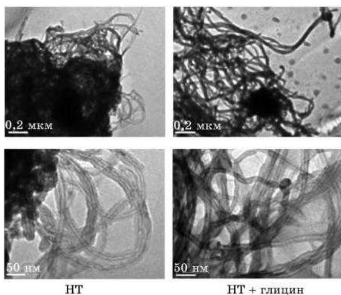
Рис. 5. ПЭМ-изображения НТ и комплекса НТ + глицин при \text{pH} = 6,0 .
