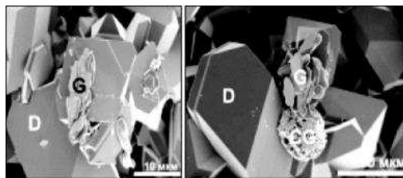
Рис. 13. Мікрофотографія зразка, одержаного з нафталіну при P = 8 \text{ ГПа} і T = 1280^\circ\text{C} : D — алмаз, G — графіт, CG — ґлобула вуглецю [60].
