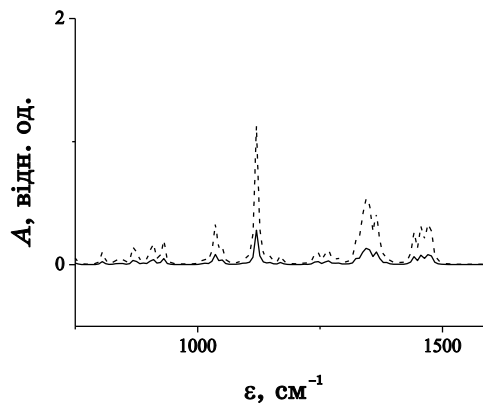
Рис. 1. Порівняння результатів розрахунку спектрів ІЧ-поглинання \gamma -коніцеїну у воді з використанням методів Гартрі–Фока (пунктирна крива) і функціонала густини (суцільна крива).
