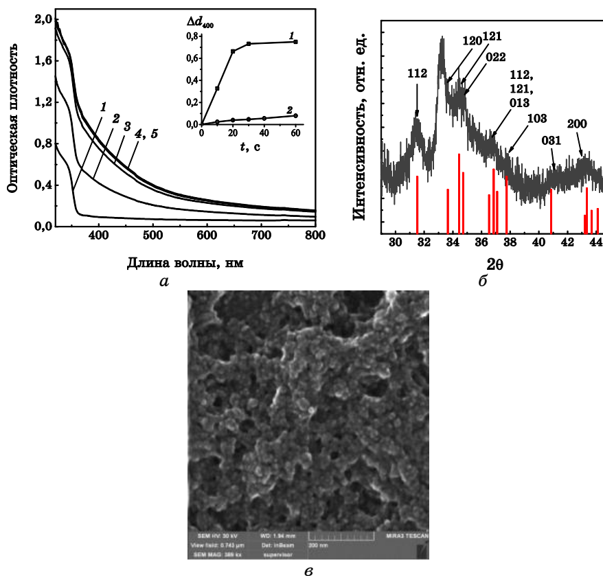
Рис. 1. а ) Спектры поглощения этанольного раствора, содержащего НЧ ZnO, AgNO 3 и S 8 до облучения (кривая 1) и после облучения на протяжении 10 (2), 20 (3), 30 (4) и 60 с (5). На вставке: изменение оптической плотности раствора при \lambda = 400 нм при облучении в присутствии НЧ ZnO (кривая 1) и в их отсутствие (2). б ) Дифрактограмма остатка, полученного испарением растворителя из облучённых в присутствии нитрата серебра и серы коллоидных растворов ZnO. Цифрами указаны индексы граней, которым принадлежат соответствующие рефлексy. Отнесение выполнено с использованием международной базы дифракционных данных (карта для акантита AgS — ICDD №01-089-3840). в ) Растровая электронная микрофотография плёнки ZnO/Ag 2 S на проводящем стекле FTO. Условия: [ZnO] = 1 \cdot 10^{-3} моль/л, [AgNO 3 ] = 3 \cdot 10^{-4} моль/л, [S 0 ] = 5 \cdot 10^{-4} моль/л.
