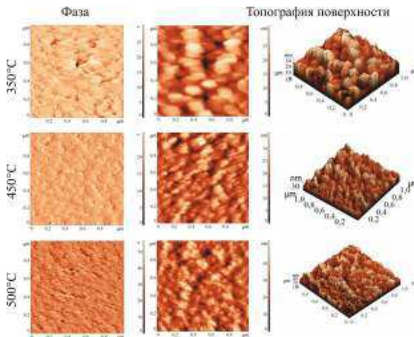
Рис. 3. АСМ-изображения ZnO:Al-плёнок (1×1 мкм) на основе изопропилового спирта в зависимости от температуры отжига, полученных золь-гель-методом на поверхности монокристаллического кремния: a — фаза, б — топография, в — трёхмерное изображение.
