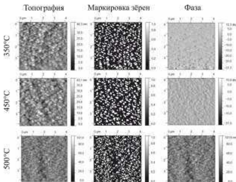
Рис. 4. АСМ-изображения ZnO:Al-плёнок (4×4 мкм) на основе изопропилового спирта в зависимости от температуры отжига, полученных золь-гель-методом на поверхности монокристаллического кремния.
