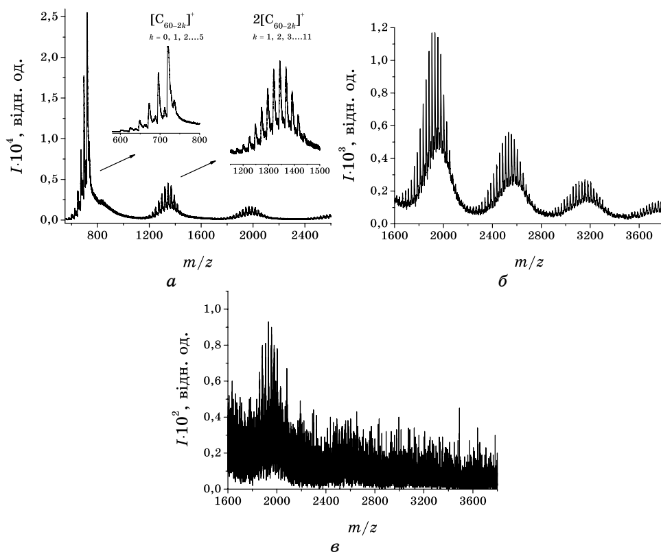
Рис. 2. Мас-спектер позитивних йонів з високим відділенням зразка C_{60}/NMP (а), одержаних при 110 \text{ мДж/см}^{-2} (б) та при 70 \text{ мДж/см}^{-2} (в) лазерного опромінення. Вставки відображають частину мас-спектру для фрагментів [C_{60-2k}]^+ , де k = 1, 2, \dots, 6 та фрагментів димера 2 \cdot [C_{60-2k}]^+ .
