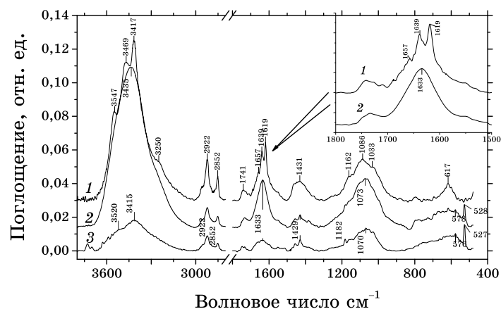
Рис. 9. ИК-фурье спектры препарата Кониум (1), фуллерена (3) и комплекса Кониума с фуллереном (2).
