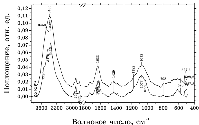
Рис. 10. ИК-спектры комплекса фуллерена с препаратом Кониум в разных концентрациях: 0,2 мл C_{60} + 0,05 мл Кониума (1), 0,2 мл C_{60} + 0,1 мл Кониума (2), 0,2 мл C_{60} + 0,2 мл Кониума (3).
