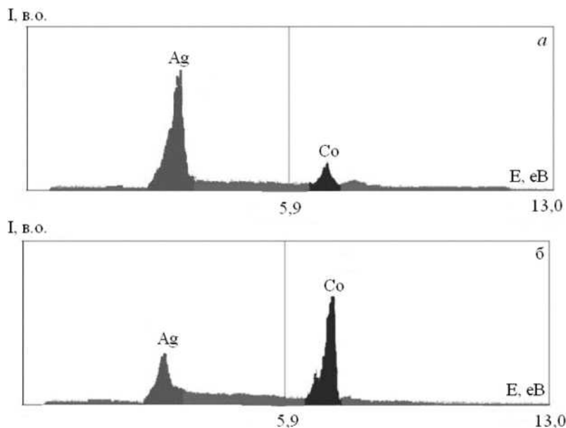
Рис. 4. Енергодисперсійні спектри від плівкових зразків Ag(35)/Co(12)/П (а) та Ag(14) + Co(28)/П (б) з ефективною концентрацією атомів Co 25 ат. % (а) і 73 ат. % (б).
