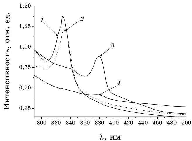
Рис. 2. Спектры поглощения мезоморфных стекловидных нанокомпозитов в системах \text{Cd}, M | \text{C}_5\text{H}_{11}\text{COO} (эквимольярного состава), допированных наночастицами сульфида кадмия (содержание CdS — 1 мол.%): 1 — M = \text{Mg}^{2+} , 2 — \text{Pb}^{2+} , 3 — \text{Sr}^{2+} .
