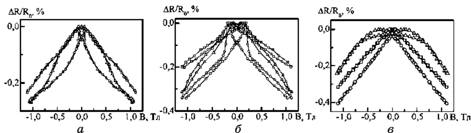
Рис. 2. Зависимость МС для [\text{Pd}(1,1)/\text{Fe}(0,9)]_3/\Pi (а), [\text{Pd}(1,1)/\text{Fe}(0,9)]_5/\Pi (б) и [\text{Pd}(1,1)/\text{Fe}(0,9)]_{10}/\Pi (в) после термического отжига до T = 780 К. Обозначения такие же, как на рис. 1.
