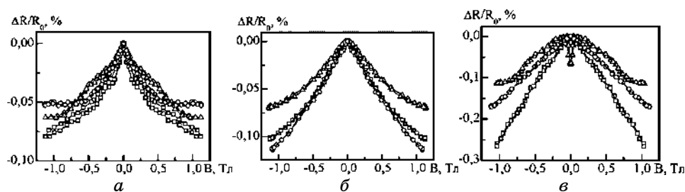
Рис. 1. Зависимость МС для [\text{Pd}(1,1)/\text{Fe}(0,9)]_3/\Pi (а), [\text{Pd}(1,1)/\text{Fe}(0,9)]_5/\Pi (б) и [\text{Pd}(1,1)/\text{Fe}(0,9)]_{10}/\Pi (в). Геометрия измерений: перпендикулярная ( \Delta ), параллельная ( \square ) и поперечная ( \diamond ).
