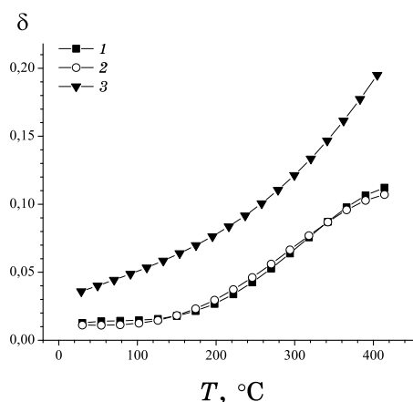
Рис. 5. Изменение ЛД на уровне \varepsilon = 2 \cdot 10^{-4} при нагреве конденсатов никеля с зерном 0,2 мкм — (1), 0,8 мкм — (2) и наноструктурированной меди [11] — (3).
