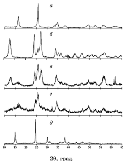
Рис. 1. Рентгенограммы порошков жёлтой \text{WO}_3 \cdot \text{H}_2\text{O} (а) и белой \text{WO}_3 \cdot 2\text{H}_2\text{O} (б) вольфрамовых кислот, а также осадков на стекле из водных сернокислых растворов \text{Na}_2\text{WO}_4 с \text{pH} = 1 (в), 3 (г) и 6 (д).
