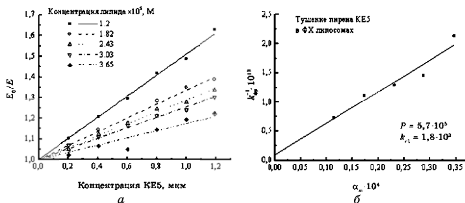
Рис. 3. Тушение флуоресценции пирена хелатом европия КЕ5 в ФХ липосомах (а) и зависимость кажущейся константы тушения пирена от объемной фракции липидной фазы (б).
