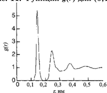
Рис. 13. Экспериментальная функция g(r) .
