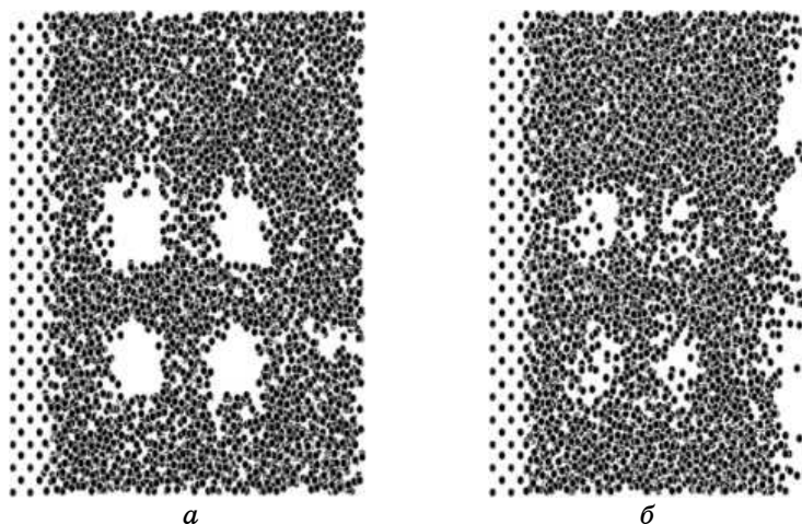
Рис. 5. Первый и последний (30000-й) шаги МД-моделирования (снимок экрана).
