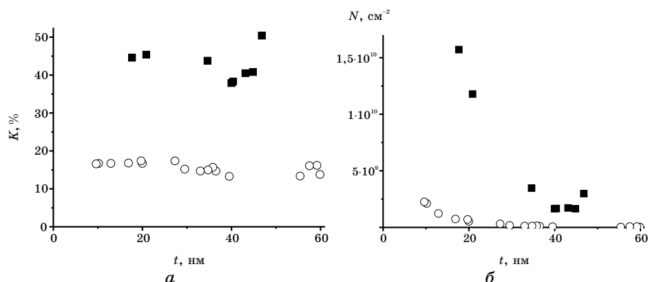
Рис. 4. Изменение с толщиной коэффициента заполнения (а) и плотности островков N (б) для систем Bi/Si (○) и Sn/Si (■).
