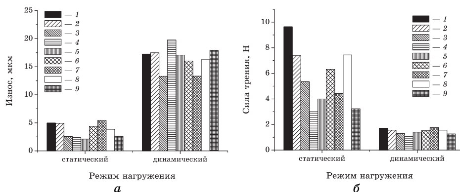
Рис. 1. Триботехнические характеристики ( a — износ; б — сила трения) смазочных композиций на основе масла И-20: 1 — базовое масло И-20; 2 — с добавками микронного порошка 2\text{H-MoS}_2 ; 3 — нанокристаллического 2\text{H-MoS}_2 ( a = 0,3136(1) нм, c = 1,257(1) нм, d_{[013]} = 3,1(2) нм; d_{[110]} = 11,3(7) нм); 4 — 1% смеси углеродных нанотрубок и указанного нанокристаллического 2\text{H-MoS}_2 ; 5 — 2% смеси углеродных нанотрубок и нанокристаллического 2\text{H-MoS}_2 ; 6 — 1% углеродных нанотрубок; 7 — 2% углеродных нанотрубок; 8 — нанокристаллического 2\text{H-WS}_2 ( a = 0,3136(1) нм, c = 1,257(1) нм, d_{[013]} = 3,1(2) нм; d_{[110]} = 11,3(7) нм); 9 — 1% смеси углеродных нанотрубок и указанного нанокристаллического 2\text{H-WS}_2 .
