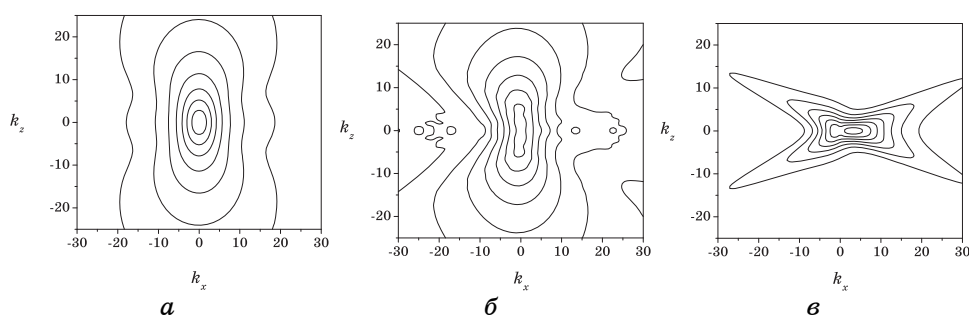
Рис. 6. Карта розподілу інтенсивності ДР в площині дифракції з врахуванням вертикальної розбіжності у випадку симетричної Ляве-дифракції характеристичного випромінення \text{CuK}_\alpha для призматичних дисльокаційних петель з дискретними орієнтаціями \langle 110 \rangle і радіусом R = 0,05|\Lambda| у кристалі Si товщиною 5 мкм (а), 50 мкм (б) і 500 мкм (в). Одиниця мірювання по осях k_x і k_z складає \pi/|\Lambda| .
