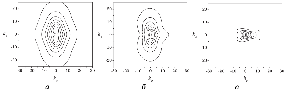
Рис. 1. Карта розподілу інтенсивності ДР в площині дифракції у випадку симетричної Ляве-дифракції характеристичного випромінювання \text{CuK}_\alpha для призматичних дислокаційних петель з дискретними орієнтаціями \langle 110 \rangle і радіусом R = 0,05|\Lambda| ( \Lambda — довжина екстинкції «сильних» Бреґгових хвиль) у кристалі Si товщиною 5 мкм (а), 50 мкм (б) і 500 мкм (в). Одиниця мірювання по осях k_x і k_z складає \pi/|\Lambda| .
