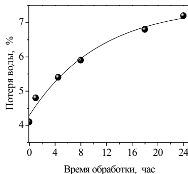
Рис. 3. Зависимость количества выделенной воды при прокаливании нанокремнезёма до 1270 К от времени механической обработки.
