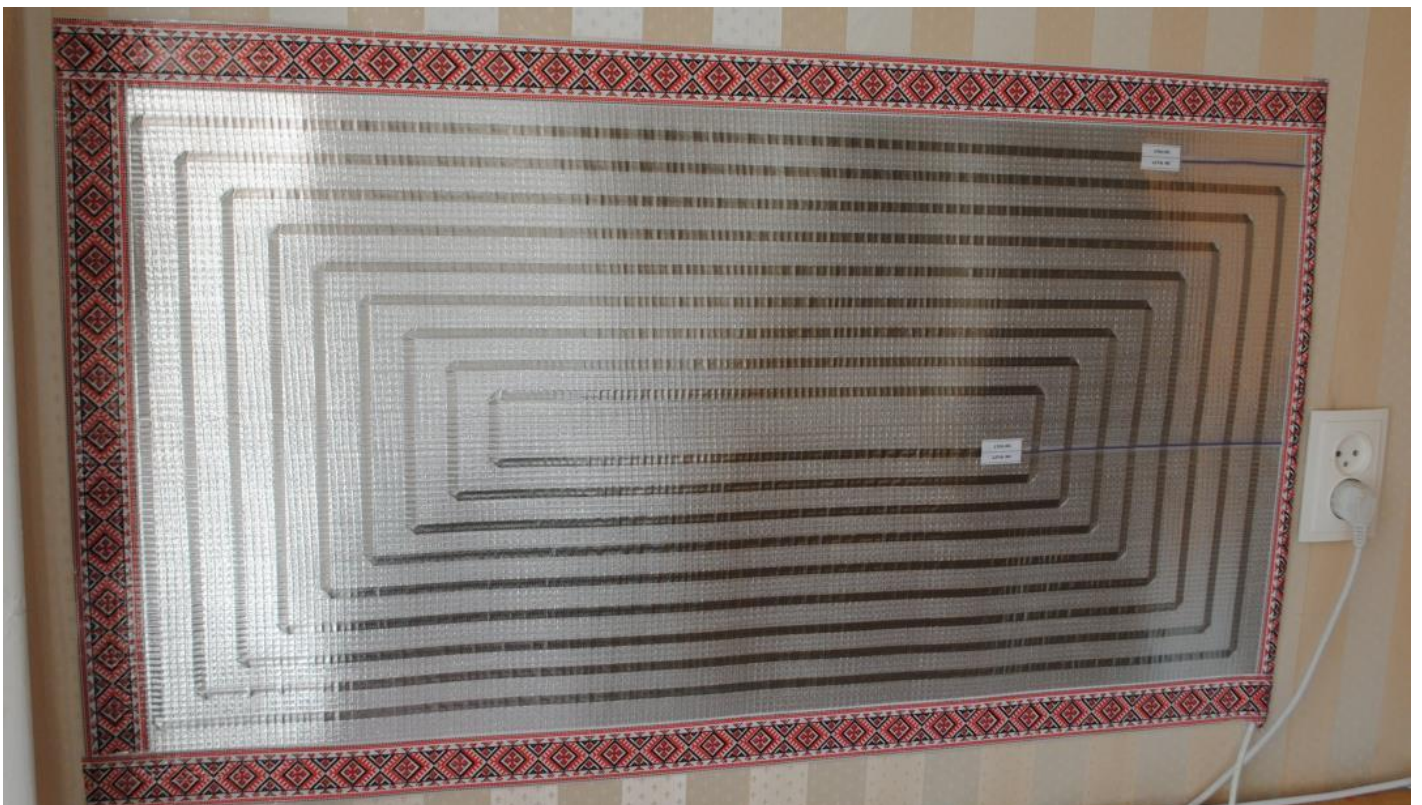
Плівковий нагрівач потужністю 250 Вт, прикріплений до стіни жилого приміщення.
